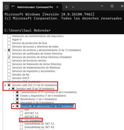
Ilustración 7 Instalación del módulo CGI
