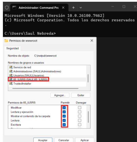
Ilustración 19 Asignar mismos permisos a los usuarios
