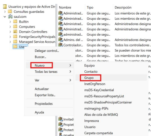
Ilustración 1 Creación de un grupo
