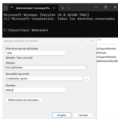
Ilustración 11 Ingreso de datos del modulo
